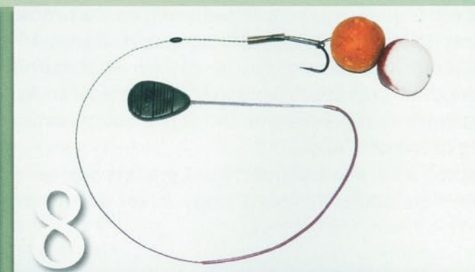
8 A gumicsövet húzzuk rá a gumistoppere, és állítsuk be az előke nyúlási hosszát.
