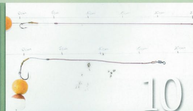
10 A kész szerelék kb. 15-17 cm zsugorítva, valós nyújtott állapotú mérete 20-25 cm.
